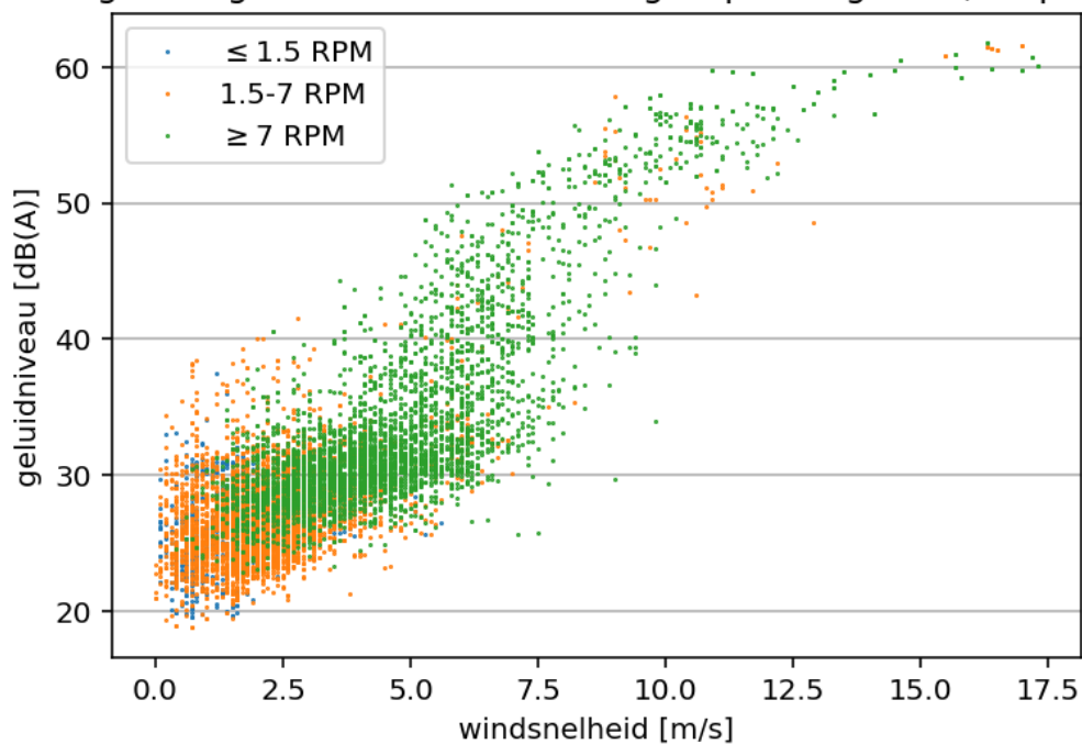
figuur 43: spreidingsdiagram voor de geluidniveaus in het laagfrequente gebied in de diepe nacht
