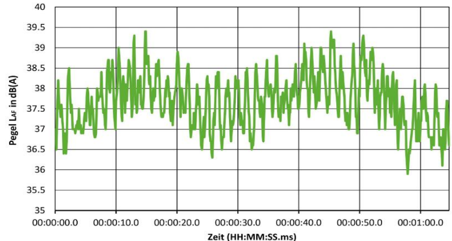
Abbildung 11: Exemplarischer Pegelschrieb bei vorliegender Amplitudenmodulation
